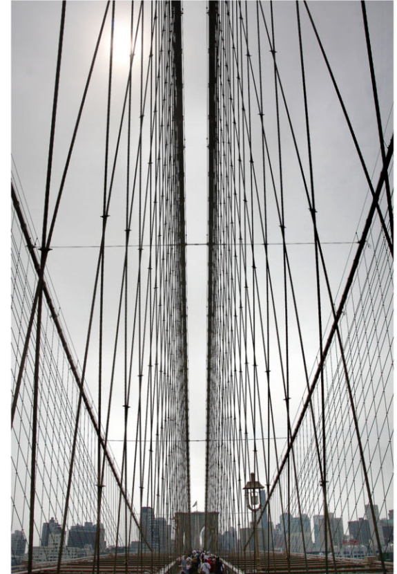
Original perspectiva del sistema de sustentación de cables del que en su día fue el puente colgante más grande del mundo, NY.
